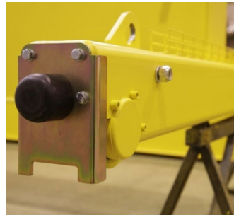
7 / Kopfträger Längsfahrt
