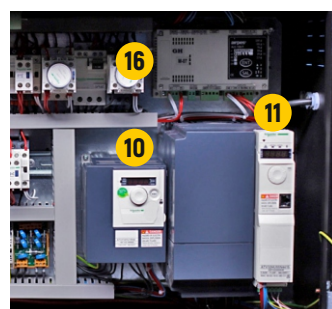
17 / Elektrischer Schaltschrank für Seilzug
