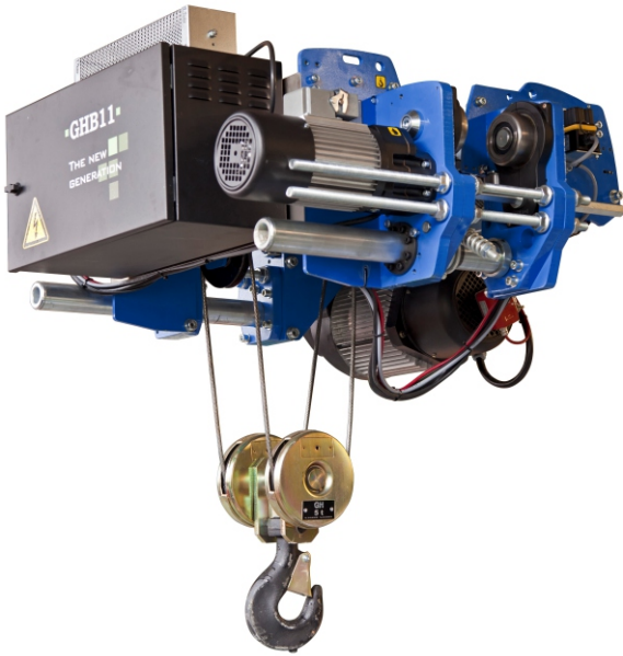
1 / Seilzug
